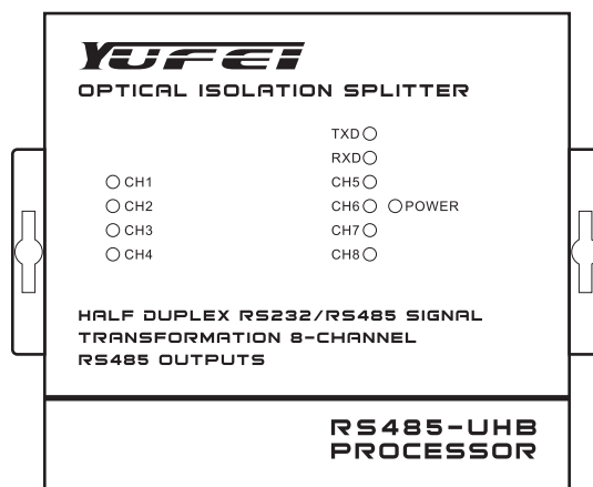
图1 YF-508D顶部面板示意图
